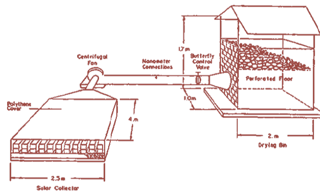
เครื่องอบแห้งด้วยแสงอาทิตย์แบบ Mixed-Type
