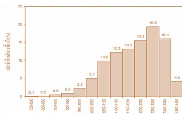
รูปแสดงการแจกแจงของรังสีตรงตามพื้นที่
