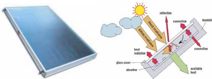
แผงรับแสงอาทิตย์แบบแผ่นเรียบ (Flat Plat Solar Collector)
