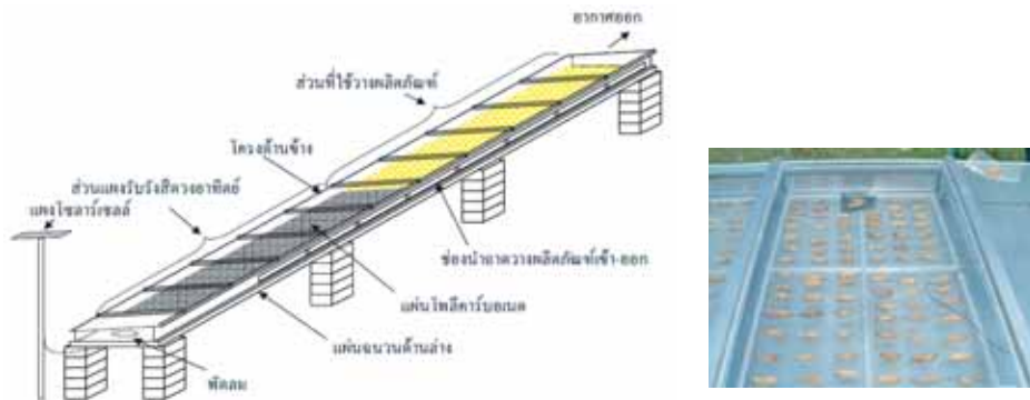
เครื่องอบแห้งพลังงานแสงอาทิตย์แบบอุโมงค์ลม
