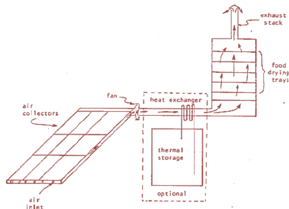
เครื่องอบแห้งด้วยแสงอาทิตย์แบบ Cabinet Dryers Fitted with Chimney and Heat Storage
