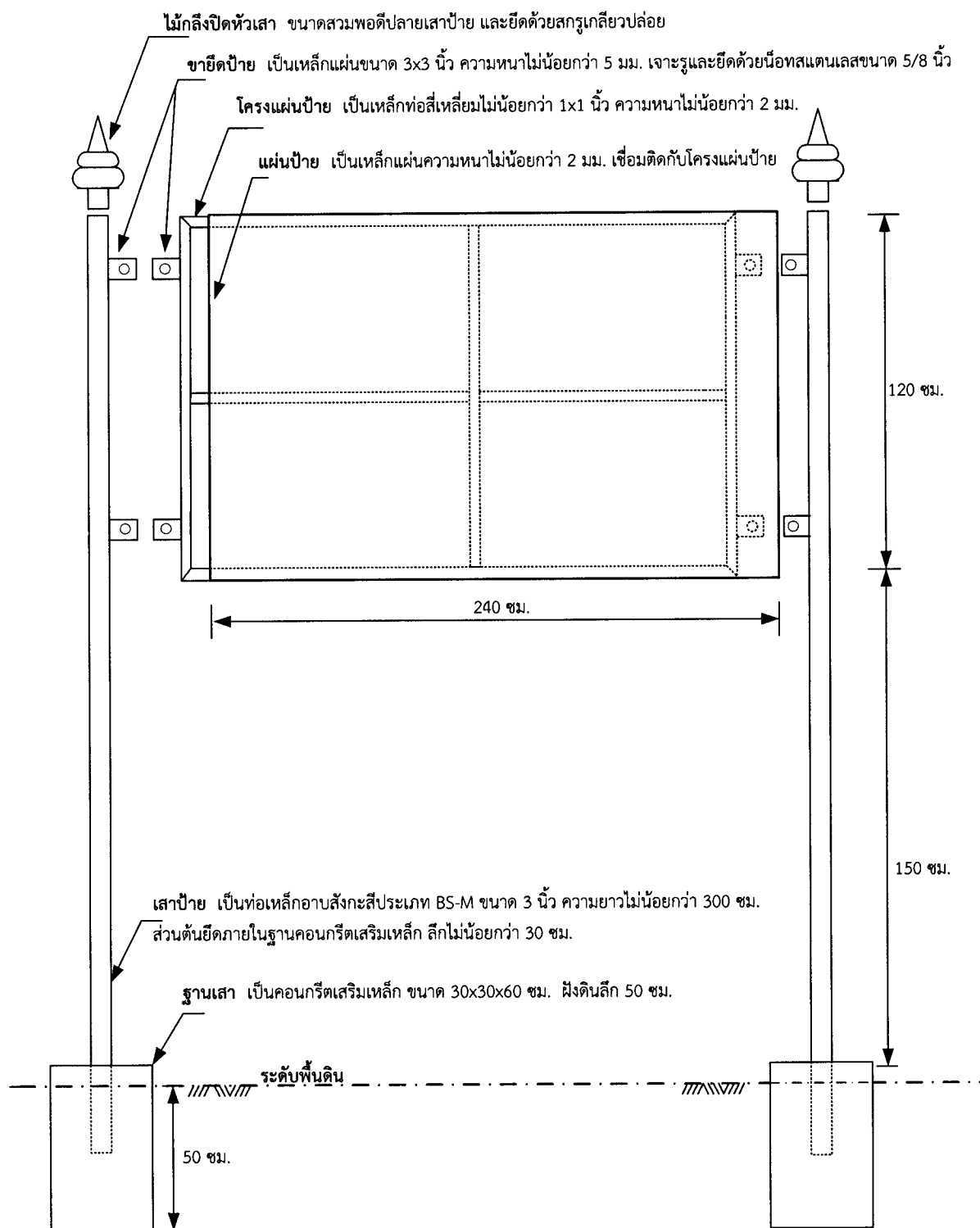
รูปที่ 3 ลักษณะรูปแบบโครงสร้างป้ายชื่อโครงการ (หมายเหตุ รูปนี้ไม่ได้แสดงอัตราส่วน)
