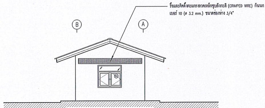
รูปด้าน 2 (เดิม)
