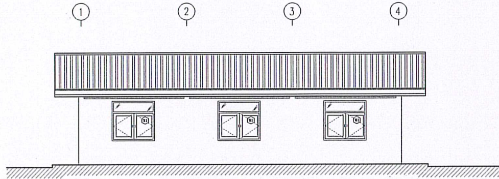
รูปด้าน 1 (เดิม) SCALE 1:100
