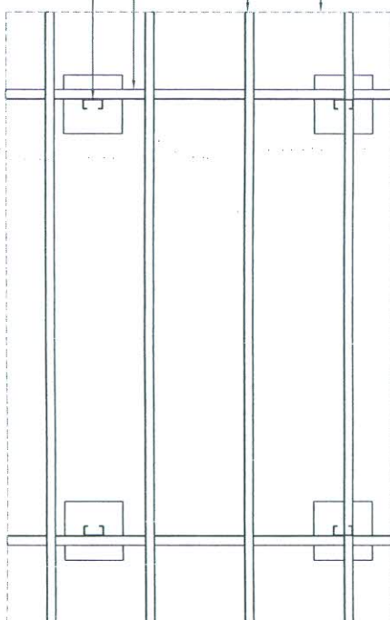
รูปด้านหน้า การติดตั้งโครงเหล็กยึดแผงเซลล์แสงอาทิตย์ มาตราส่วน 1:25
