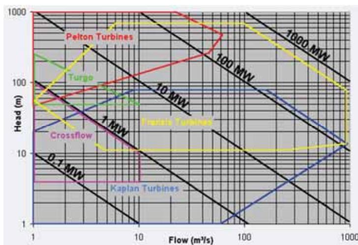
รูปแสดง Turbine Application Chart
