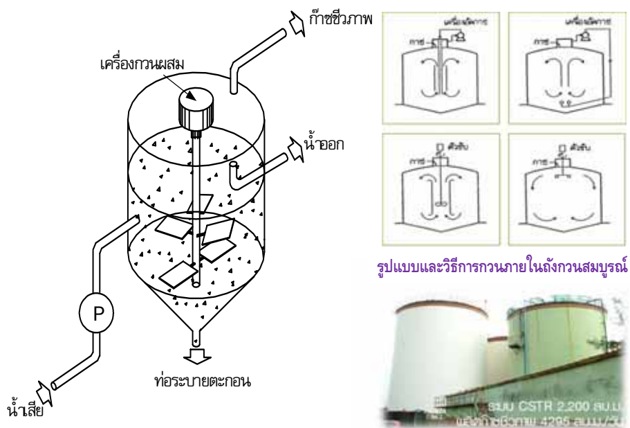
รูปแสดงระบบผลิตก๊าซชีวภาพแบบถังกวนสมบูรณ์ (Completely Stirred Tank Reactor)
