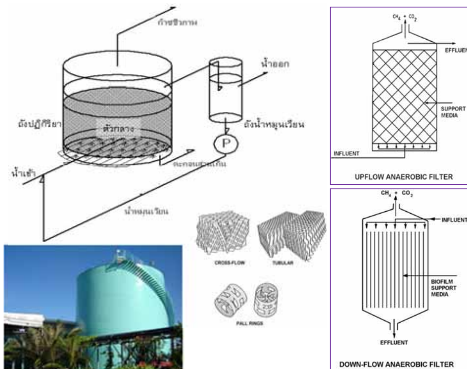
รูปแสดงลักษณะของระบบผลิตก๊าซชีวภาพแบบ Anaerobic Fixed Film or Anaerobic Filter
