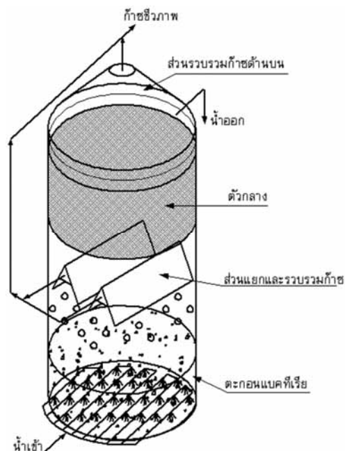
รูปแสดงลักษณะของระบบผลิตก๊าซชีวภาพแบบ Anaerobic Hybrid Reactor
