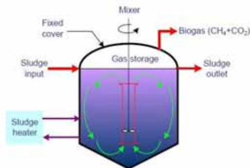
รูปแสดงลักษณะการทำงานของกลุ่บ่อหมักไร้ออกซิเจนแบบเร็ว
