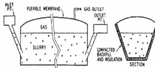
รูปแสดงบ่อหมักข้าแบบราง (Plug Flow digester)
