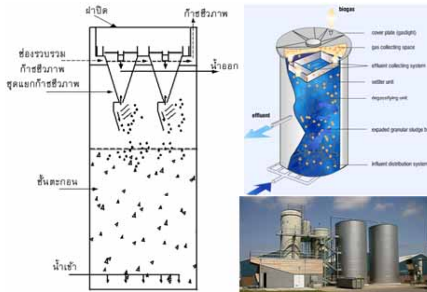
รูปแสดงลักษณะของระบบผลิตก๊าซชีวภาพแบบExtended Granular Sludge Bed
