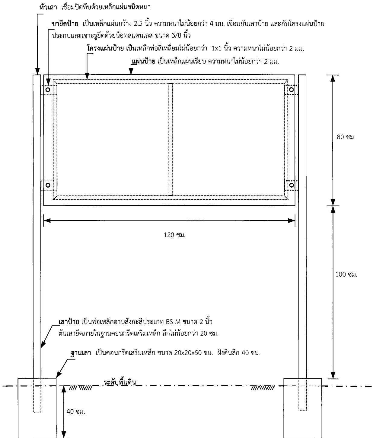
รูปที่ 3 ลักษณะป้ายแสดงข้อมูลทางเทคนิค (รูปนี้ไม่ได้แสดงอัตราส่วน)
