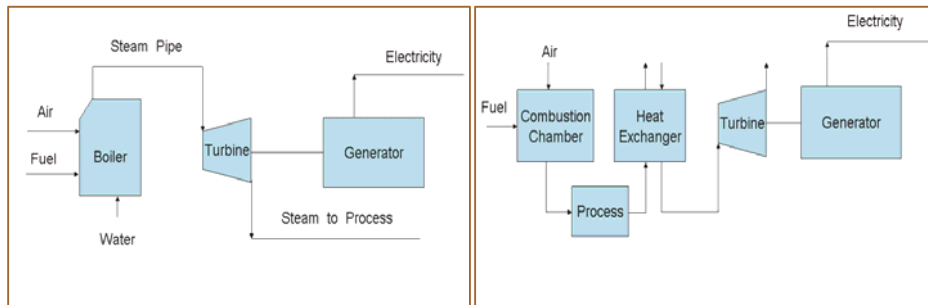
แบบการผลิตไฟฟ้าหน้า (ซ้าย) และการผลิตไฟฟ้าตามหลัง (ขวา)
