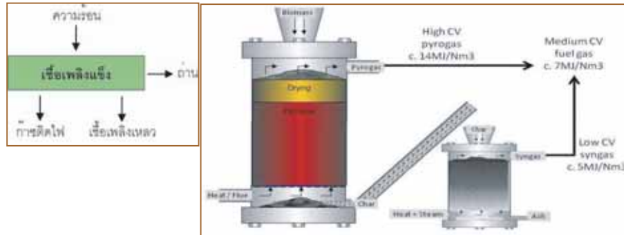
รูปแสดงกระบวนการ Pyrolysis
