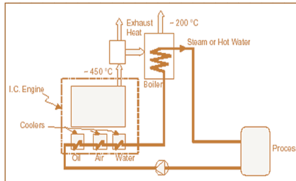
รูปแสดง Internal Combustion Engine Cogeneration
