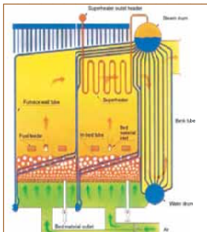
รูปแสดงลักษณะเตาเผาเชื้อเพลิงระบบฟลูอิดไคซ์เบด
