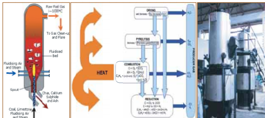
รูปแสดงกระบวนการ Gasification และเตา Gasifier
