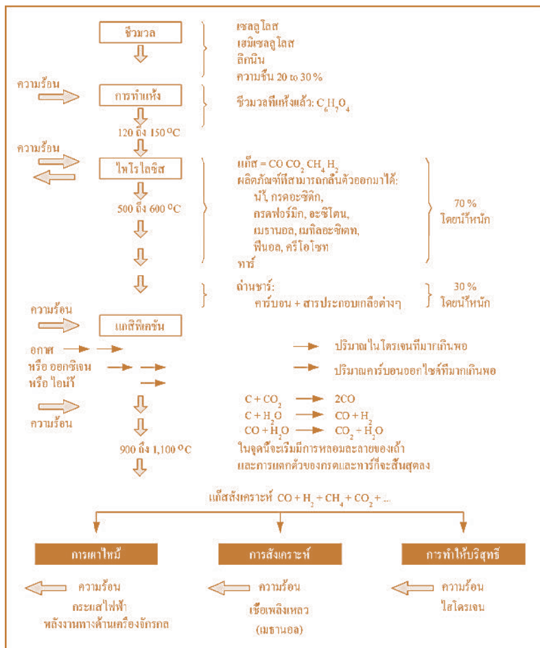
รูปแสดงกระบวนการไพโรไลซิสร่วมกับกระบวนการแก๊สซิฟิเคชัน
