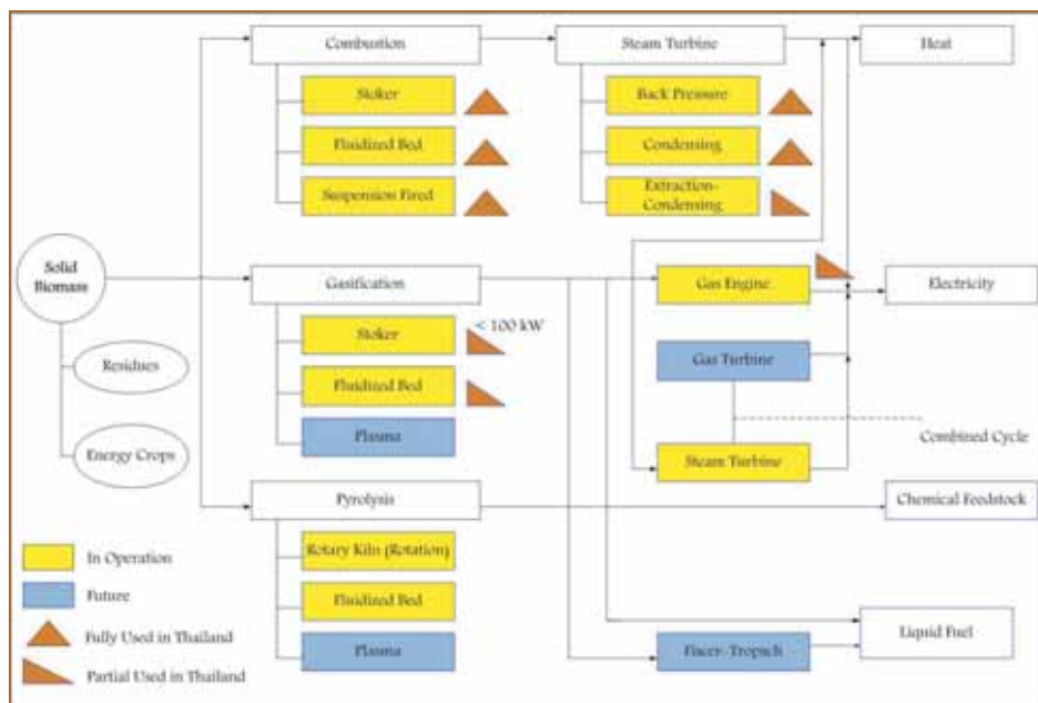
รูปแสดงเทคโนโลยีการผลิตพลังงานจากเชื้อเพลิงชีวมวล
