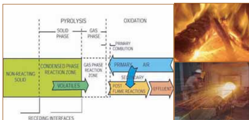
รูปแสดงการเผาไหม้โดยตรงของชีวมวล
