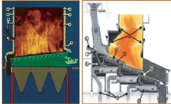
รูปแสดงลักษณะเตาเผาเชื้อเพลิงระบบสโตกเกอร์แบบกระจาย
