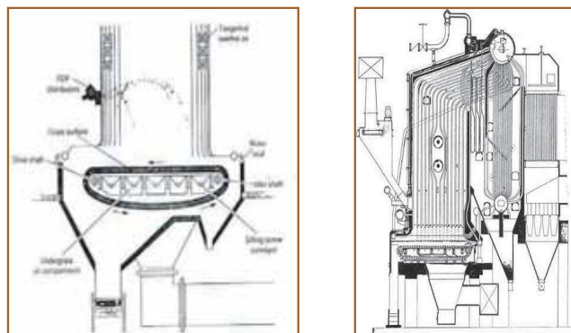
รูปแสดงลักษณะเตาเผาเชื้อเพลิงระบบสโตเกอร์แบบตะกรับเลื่อน
