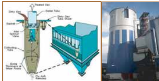
รูปแสดงไซโคลน (Cyclone)
