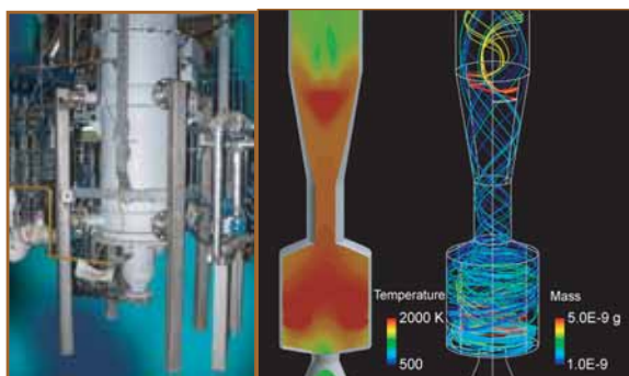
รูปแสดงเตาแบบ Entrained Bed Gasifier
