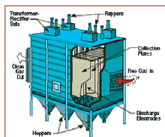
รูปแสดง Electrostatic Precipitator (ESP)
