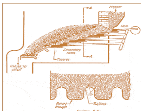
รูปแสดงลักษณะเตาเผาเชื้อเพลิงระบบสโตกเกอร์ที่เชื้อเพลิงถูกป้อนเข้าสู่เตาทางด้านล่าง
