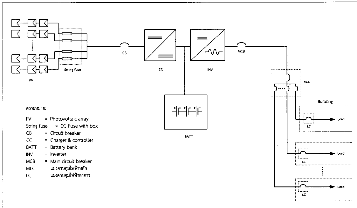
รูปที่ 1 ไตอะแกรมลักษณะระบบผลิตไฟฟ้าด้วยเซลล์แสงอาทิตย์
