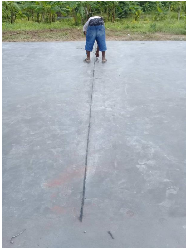
รูปที่ 20 การใส่แอสฟัลต์ผสมทรายที่แนวรอยต่อระหว่างพื้นคอนกรีต
