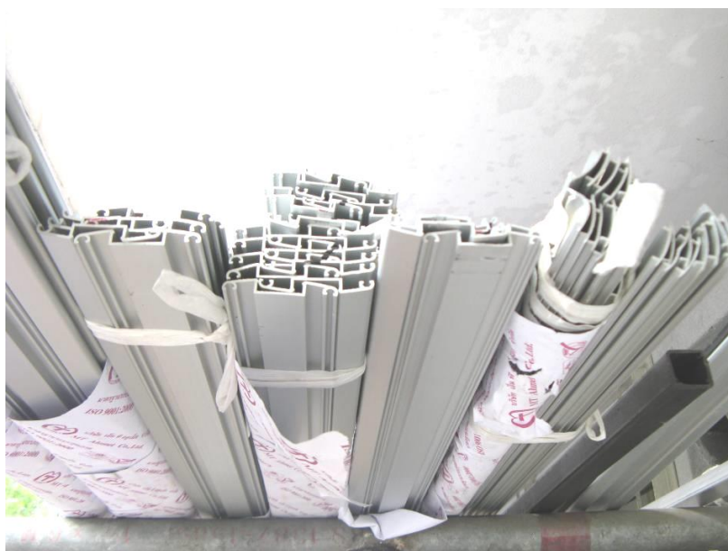
รูปที่ 35 ชุด Aluminium Clamping ที่ใช้ยึดแผ่นโพลีคาร์บอเนตกับโครงสร้างของระบบอบแห้งฯ
