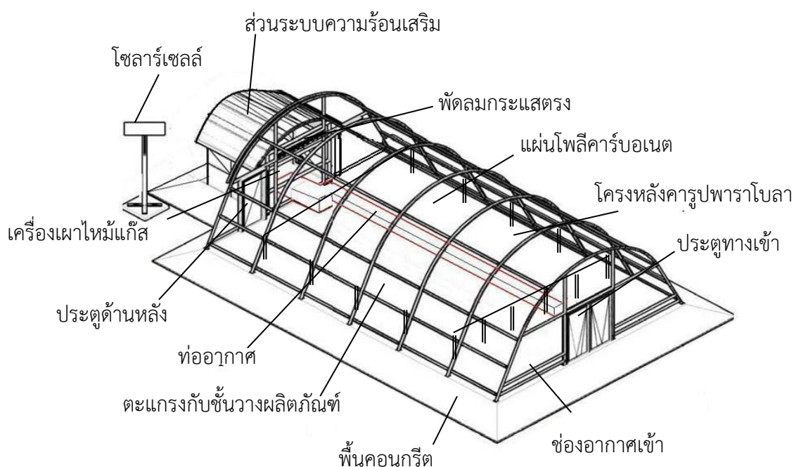
รูปที่ 1 โครงสร้างและส่วนประกอบระบบอบแห้งแบบเรือนกระจก (แบบ พพ. 3)
