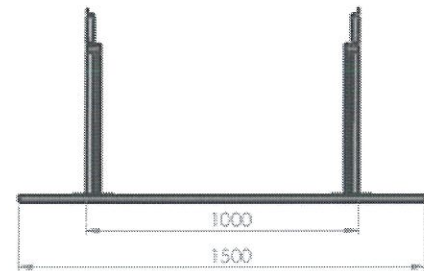
รูปมุมมองด้านหน้า Scale 1:15
