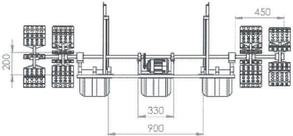
รูปมุมมองด้านหน้า Scale 1:15
