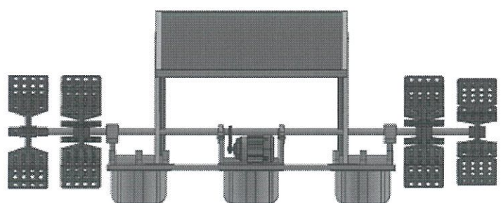
รูปมุมมองด้านหน้า Scale 1:15
