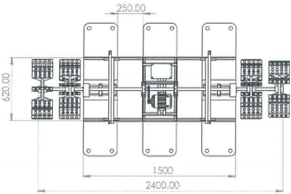
รูปมุมมองด้านบน Scale 1:15
