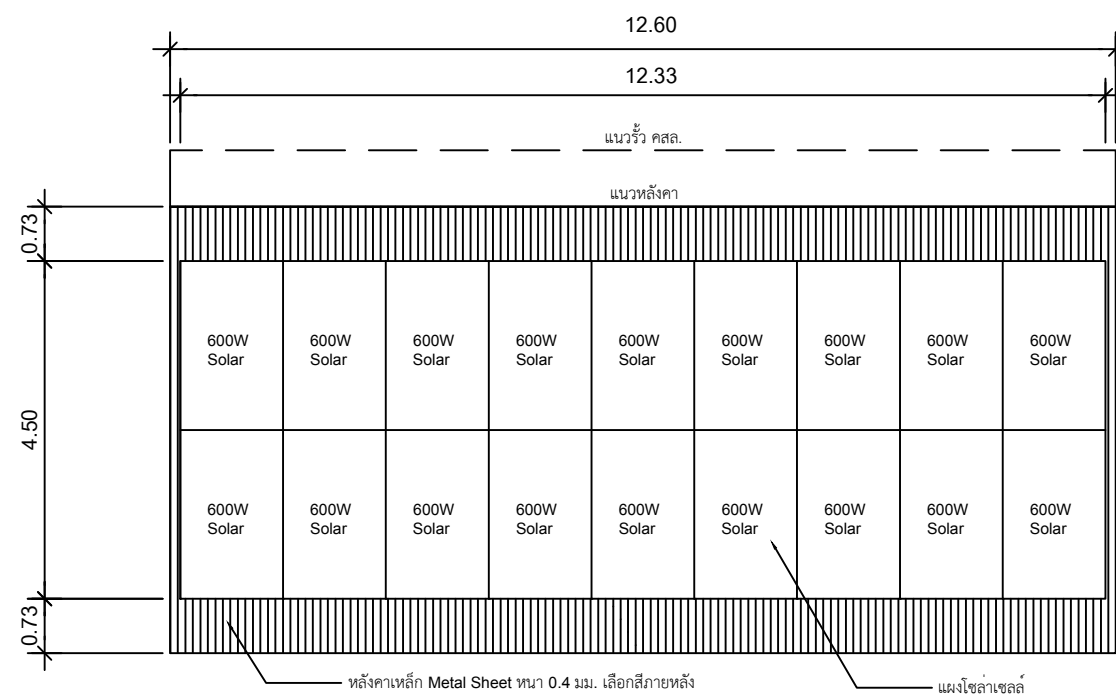
แปลนพื้นที่ติดตั้งโซลาร์เซลล์ มาตราส่วน 1 : 100
