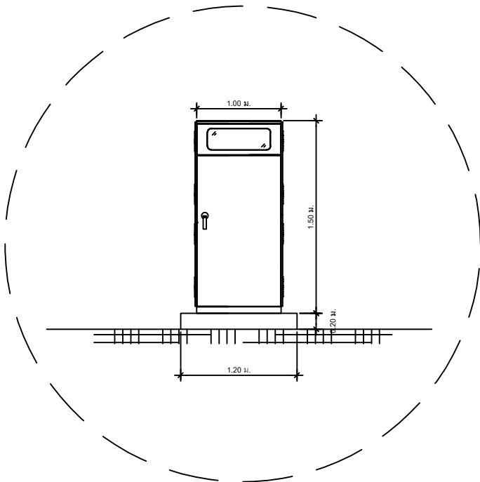
ตู้ควบคุมระบบไฟฟ้า
