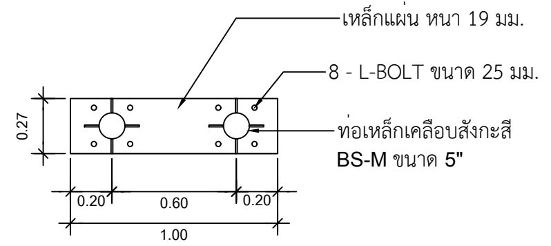
ขยาย PLATE มาตราส่วน 1 : 25
