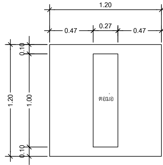
แปลนฐานราก F 1 : 25
