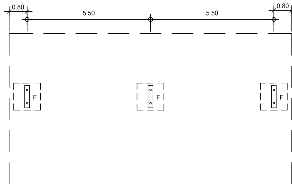
แปลนรากฐาน มาตราส่วน 1 : 100
