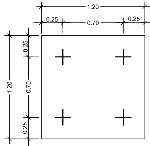
ขยายจากราก F 1 : 25
