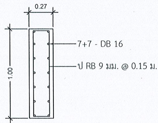
ขยายคาน มาตราส่วน 1 : 25
