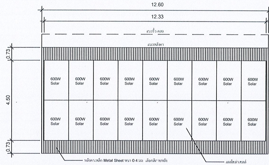
แปลนพื้นที่ติดตั้งโซลาร์เซลล์ มาตราส่วน 1 : 100
