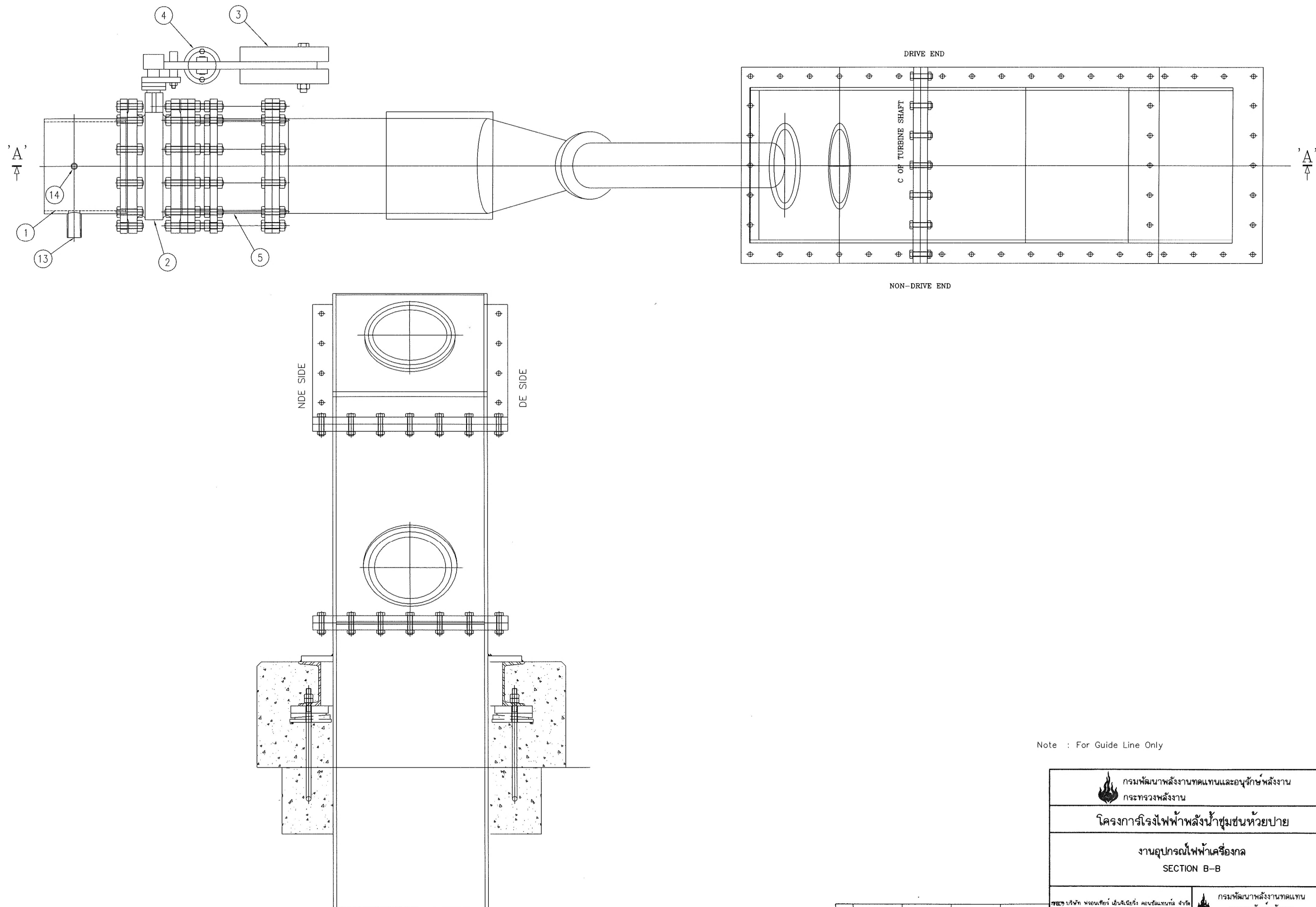
SECTION 'B' - 'B'
