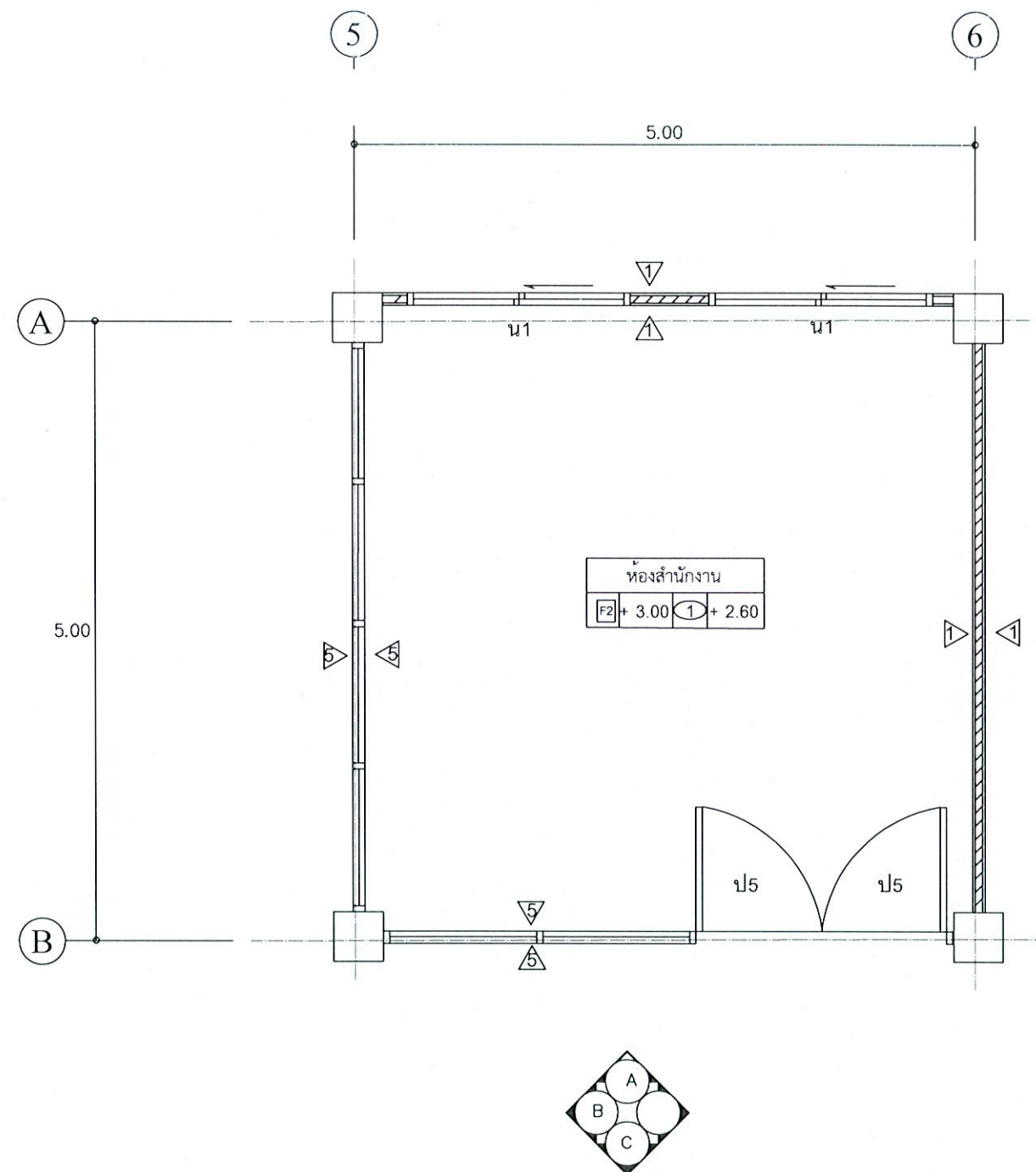
แบบขยายห้องสำนักงาน
