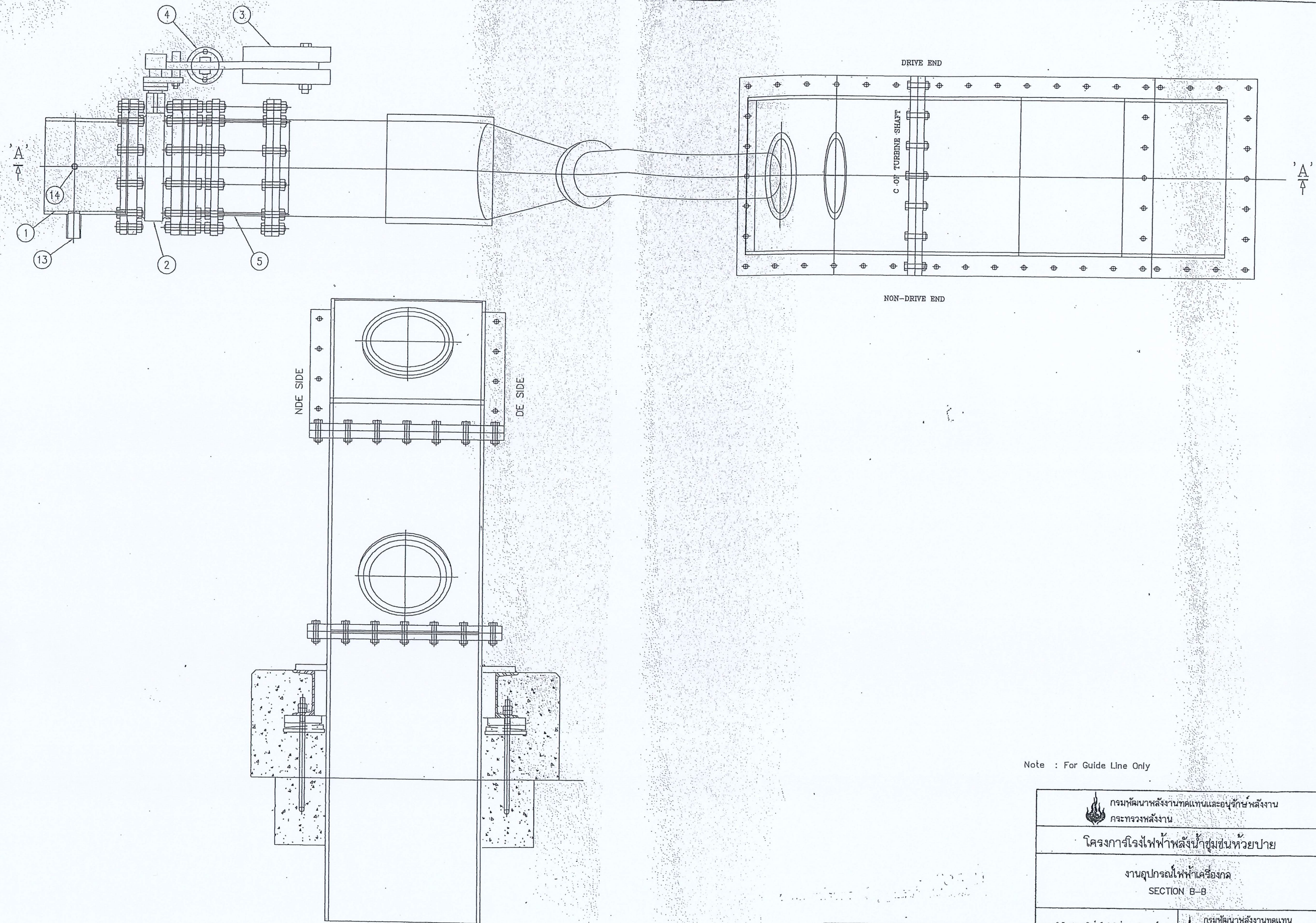
SECTION 'B'-'B'
