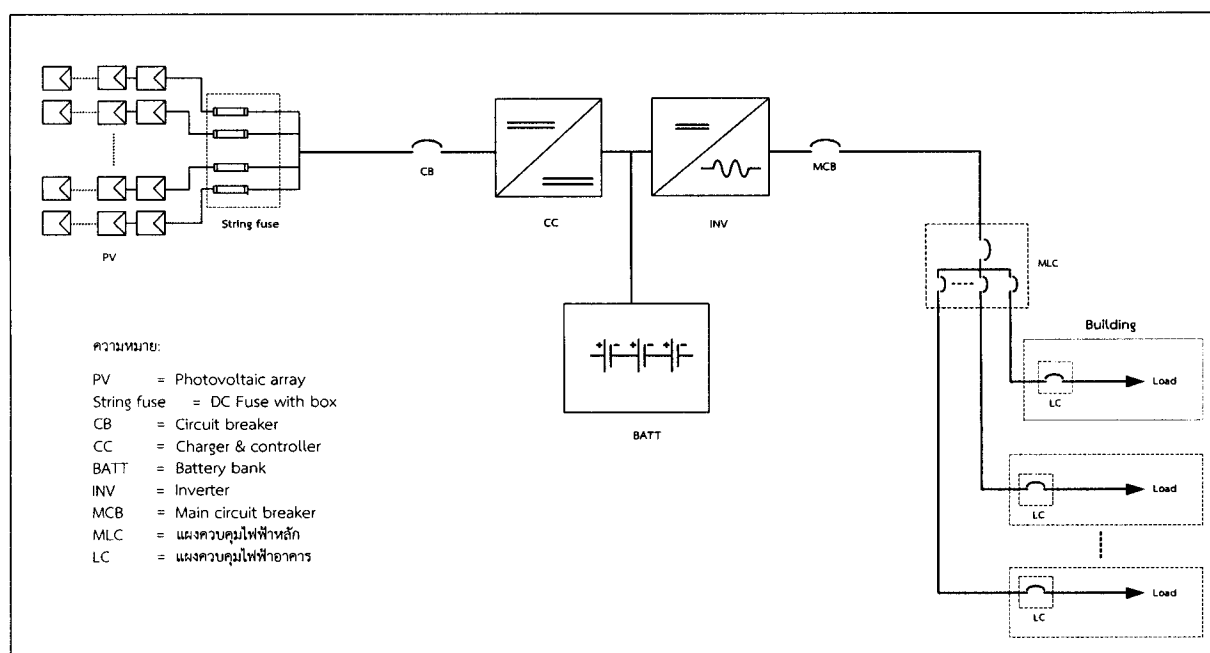
รูปที่ 1 ไดอะแกรมลักษณะระบบผลิตไฟฟ้าด้วยเซลล์แสงอาทิตย์
