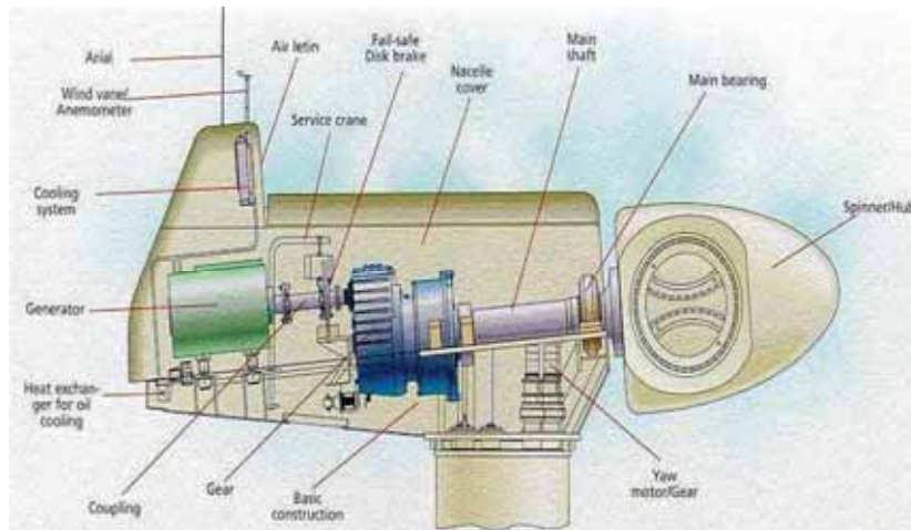
รูปแสดงส่วนประกอบภายในนาเซล
