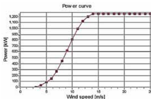
กังหันลม ขนาด 1,250 กิโลวัตต์
