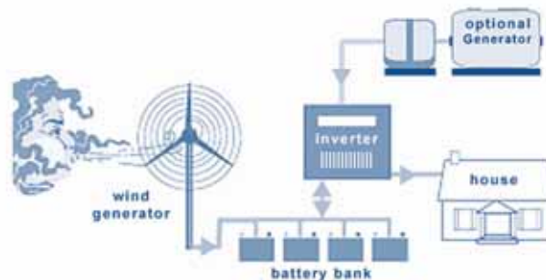
ระบบการติดตั้งใช้งานแบบเดี่ยว
