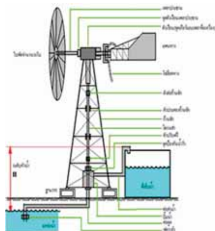
กังหันลมสูบน้ำเพื่อการเกษตรและปศุสัตว์
