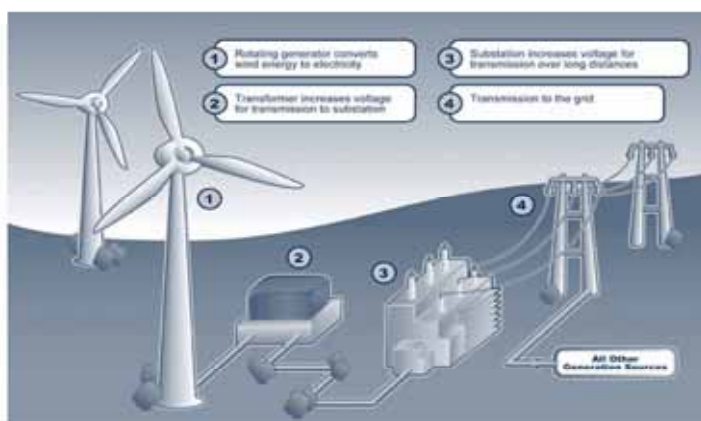
ระบบการติดตั้งใช้งานแบบเชื่อมต่อเข้าสู่ระบบสายส่ง
