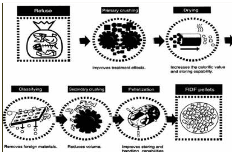
รูปแสดงขั้นตอนในการแปรรูปขยะเป็นเชื้อเพลิงขยะ
