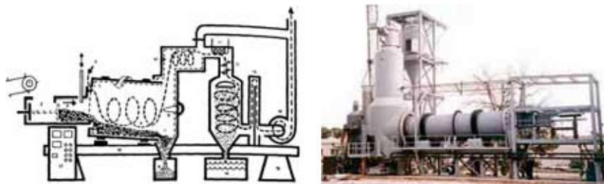
เตาเผาแบบหมุน
