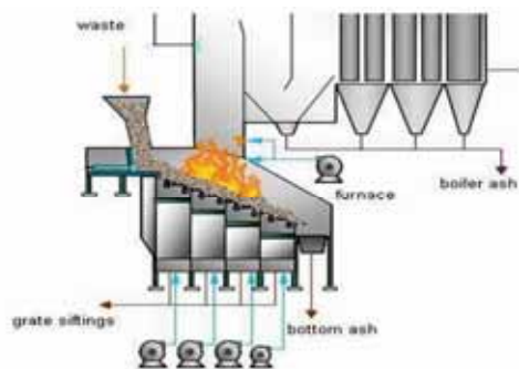
เตาเผาแบบตะกรับ
