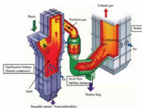
เตาเผาผลิตก๊าซเชื้อเพลิงจากขยะชุมชน
