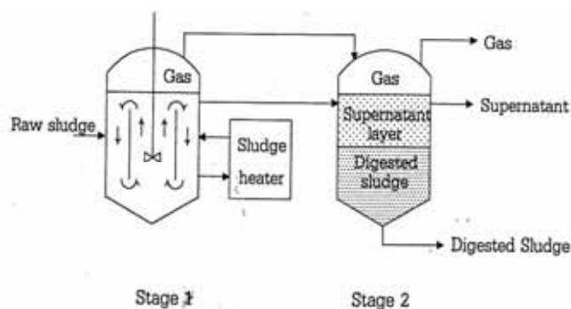
รูปแสดงถังย่อยแบบอัตราสูงที่มีการแยกตะกอน
