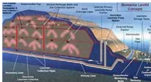
แบบ Bioreactor Landfill
