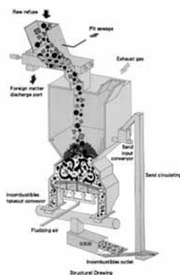
เตาเผาแบบฟลูอิดไคซ์เบด
