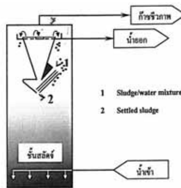
รูปภาพตัดขวางของถังหมักแบบ EGSB
