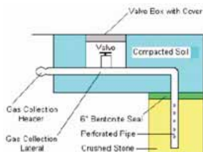
ระบบควบคุมก๊าซชีวภาพจากหลุมฝังกลบขยะมูลฝอยแบบ Active System
