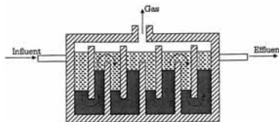
รูประบบ Anaerobic Baffled Reactor
