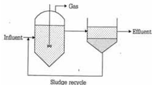
รูปแสดงถังย่อยแบบสัมผัส
