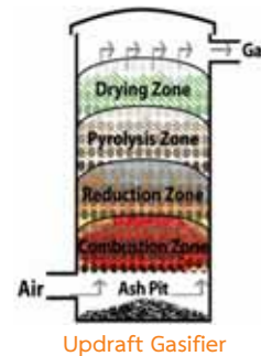
Updraft Gasifier
