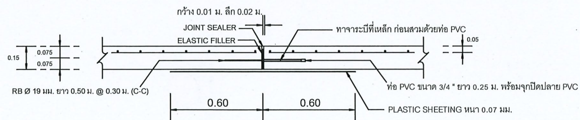
แบบขยาย EXPANTION JOINT (ทุกระยะไม่เกิน 50 ม.)
