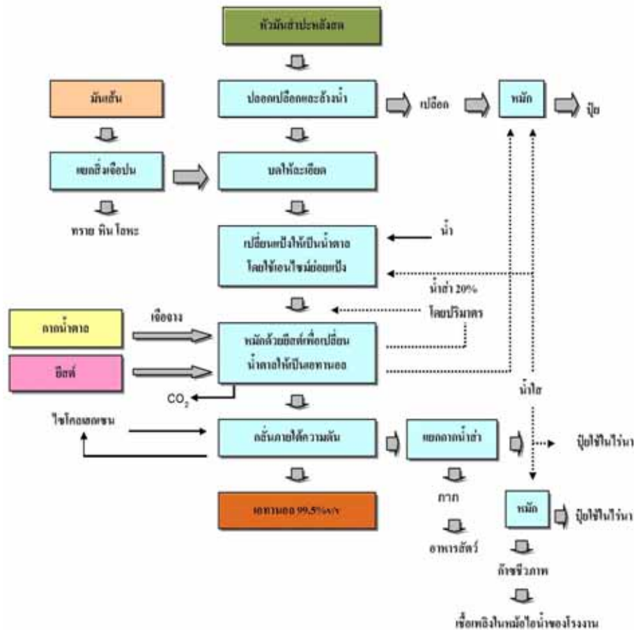
รูปแผนผังแสดงขั้นตอนการผลิตเอทานอลจากมันสำปะหลังและอ้อยในโรงงานต้นแบบของ วว.
