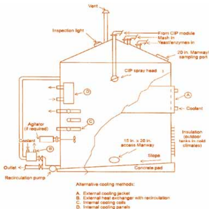
รูปแสดงถังหมักแบบ (Batch)
