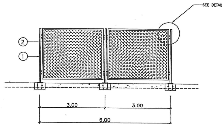
แบบรั้วตาข่ายลอมเสาวัดลม
