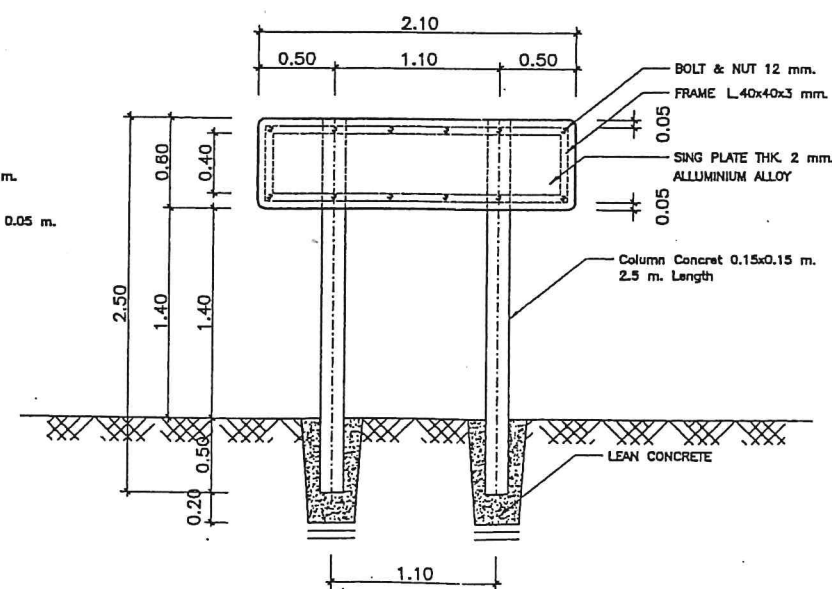
แบบขยายป้าย
