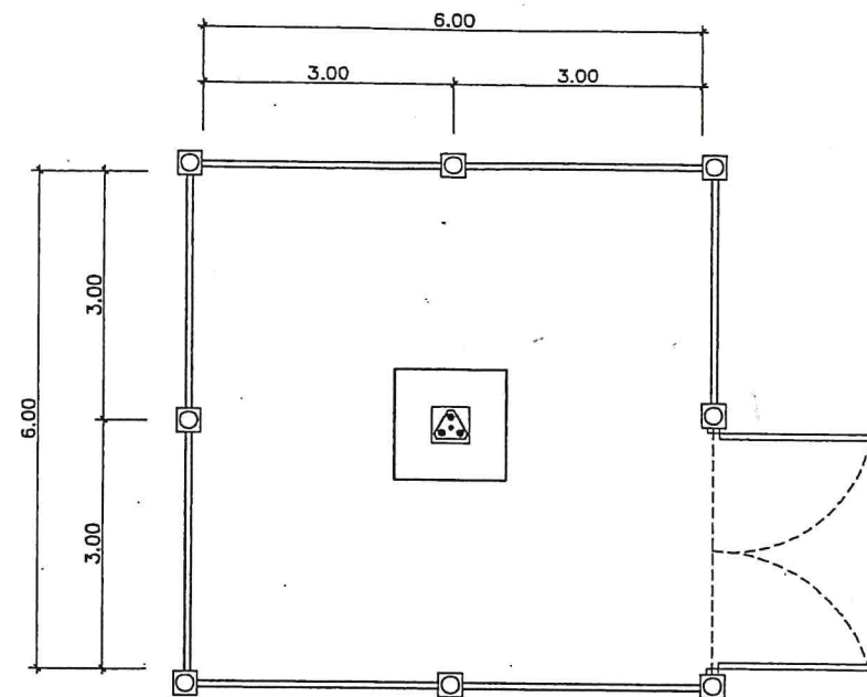
แบบรั้วตาข่ายลอมเสาวัดลม
