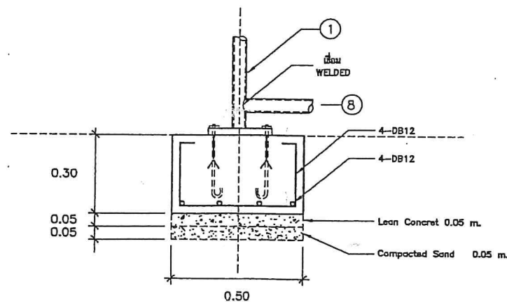
แบบแสดงฐานราก
