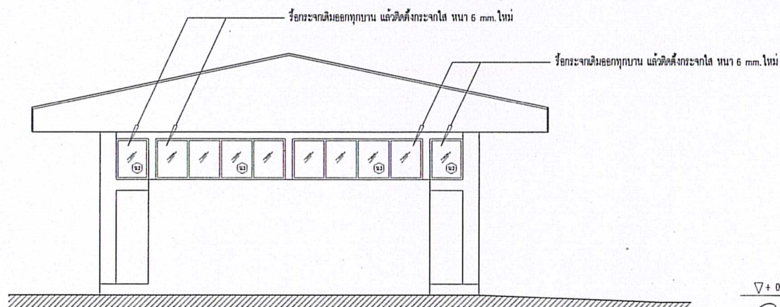
รูปด้าน A (ปรับปรุงใหม่)
