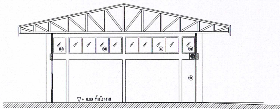
ภาพตัด 2 (เดิม)
