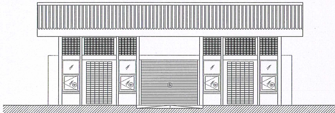
รูปด้าน D (ปรับปรุงใหม่)
